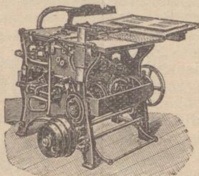
Octav-Falzmaschine für 3 Bruch mit Faden-Heftapparat zum gleichzeitigen Holländern der gefalzten Bogen.
