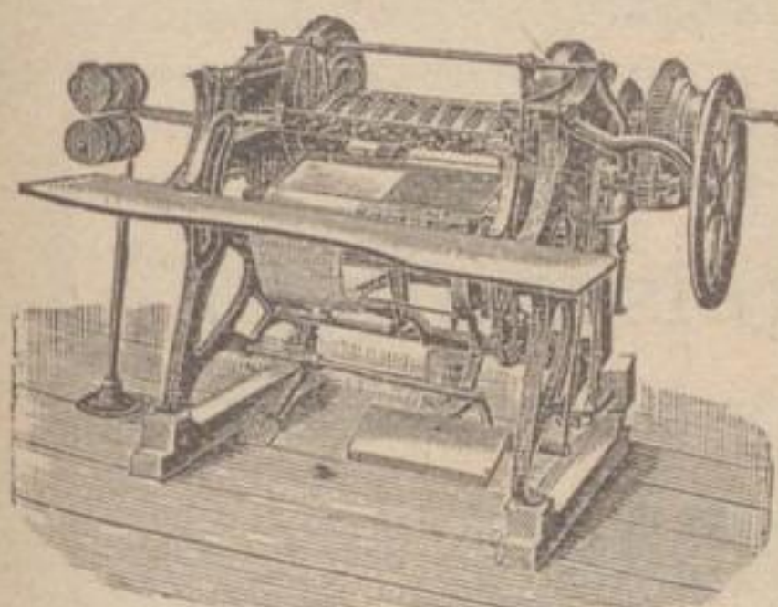
Royal Drahtbuch-Heftmaschine für Geschäftsbücher und Verlagswerke, heftet bis 52 cm Höhe und 14 cm Dicke
