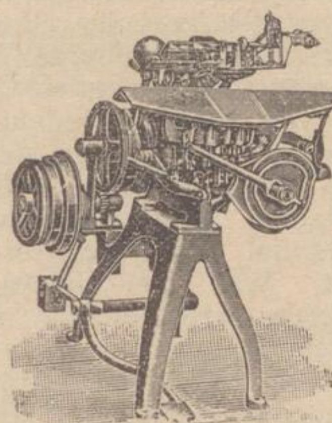
Faden-Heftmaschine für Schreib- u. Zeichen-Hefte mit selbstth. Verknotung des Fadens.
