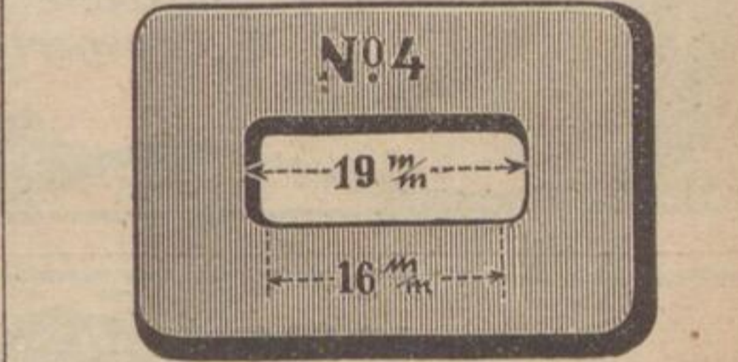
No. 4 passend für Bandeisen bis 16 mm Breite und schmalere Sorten.
