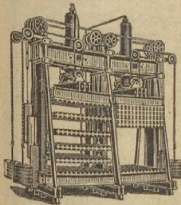
Hydraulische Spielkarten- Presse, neu.
