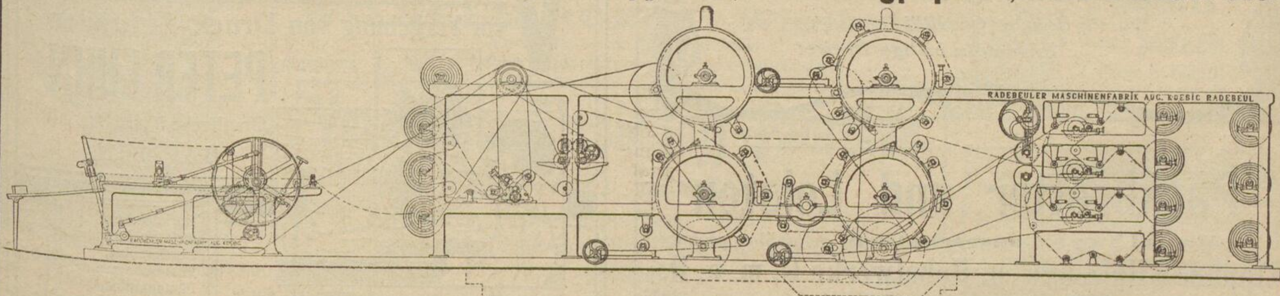
(Ansicht einer Rollenklebmaschine für 2-4 Rollen, mit Reserverollen-Gestell, mit 4 Trockencylindern, mit Anfeuchter, Aufrollvorrichtung und separat stehendem Querschneider) [144482]
