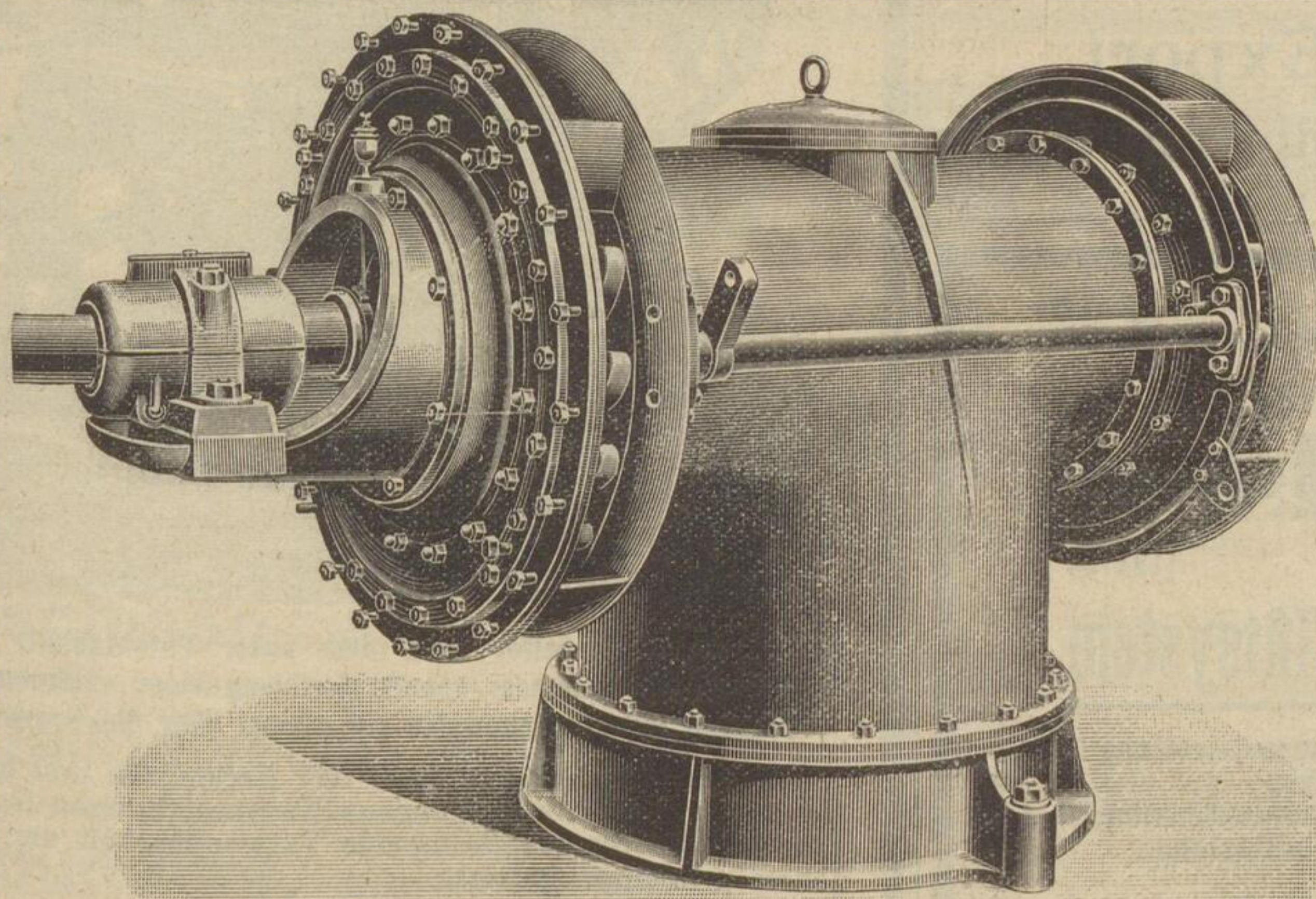
Zwillings-Francis-Turbine mit liegender Welle
