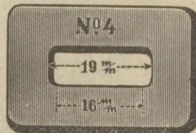
No. 4 passend für Bandeisen bis 16 mm Breite und schmalere Sorten.
