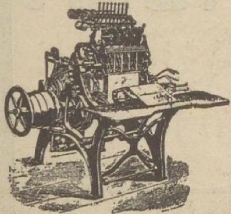
Faden-Heftmaschine „EH“ für Bücher und Broschüren ohne Einschneiden der Lagen.
