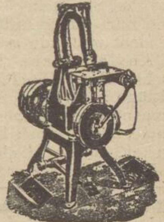
Broschüren-Heftmaschine Nr. „2 E“ für ca. 23 mm Heftstärke von beiden Seiten durch den Falz heftend.
