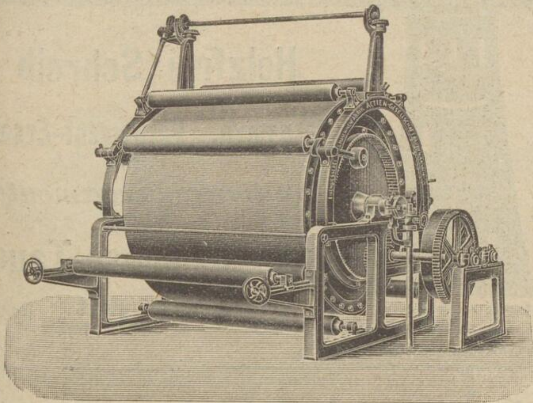
Pappentrocken-Apparat
