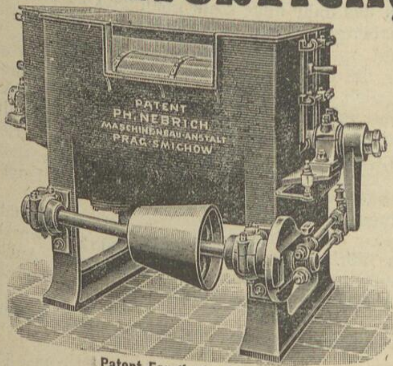
Patent-Fan-Knotenfänger
