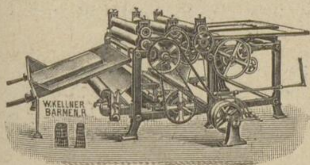
Bogen-Kaschier-Maschine
