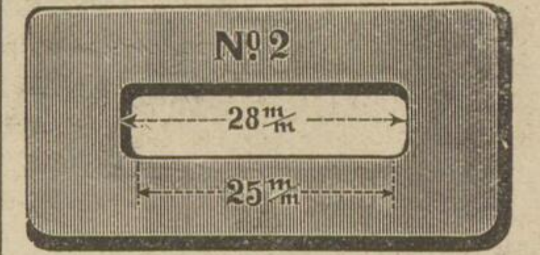
No. 2 passend für Bandeisen bis 25 mm Breite
