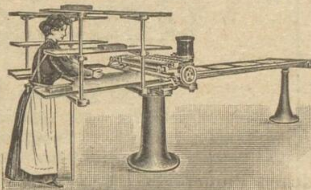
Anleimmaschine mit autom. Transport Modell „Tipp-Topp“
