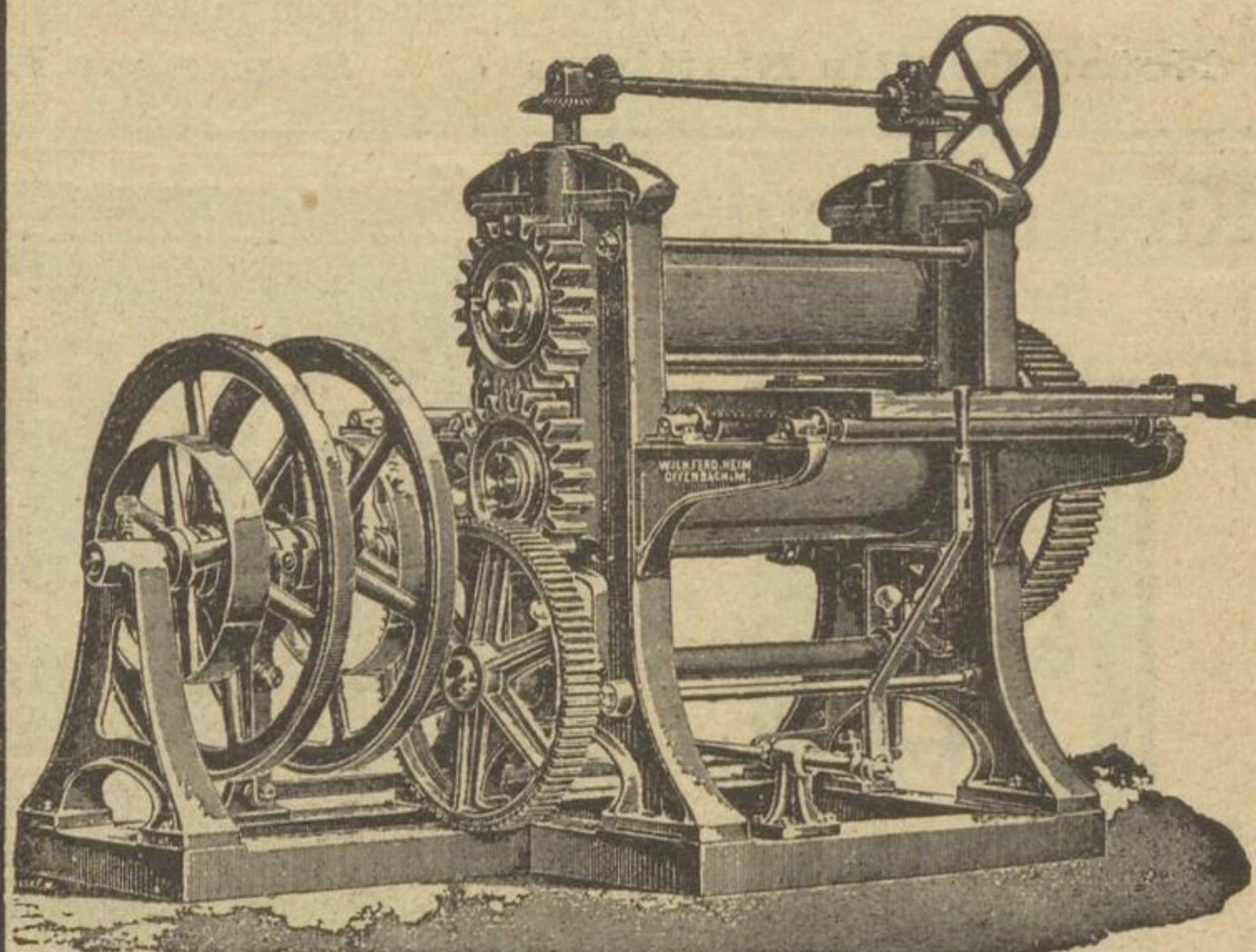
Schweres Walzwerk zum Prägen und Ausschneiden
