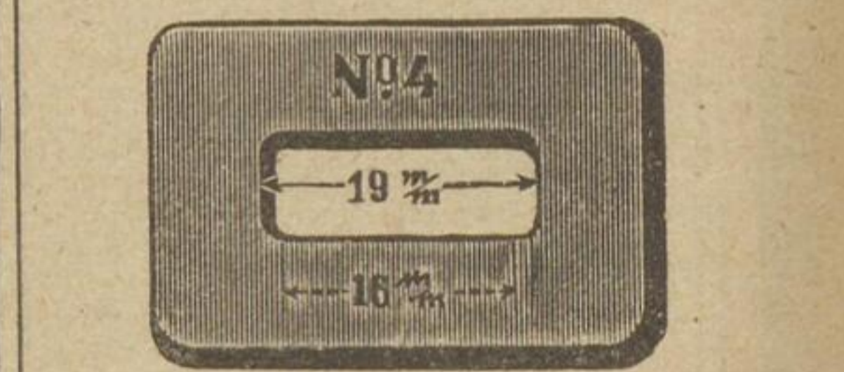
No. 4 passend für Bandeseisen bis 16 mm Breite und schmalere Sorten
