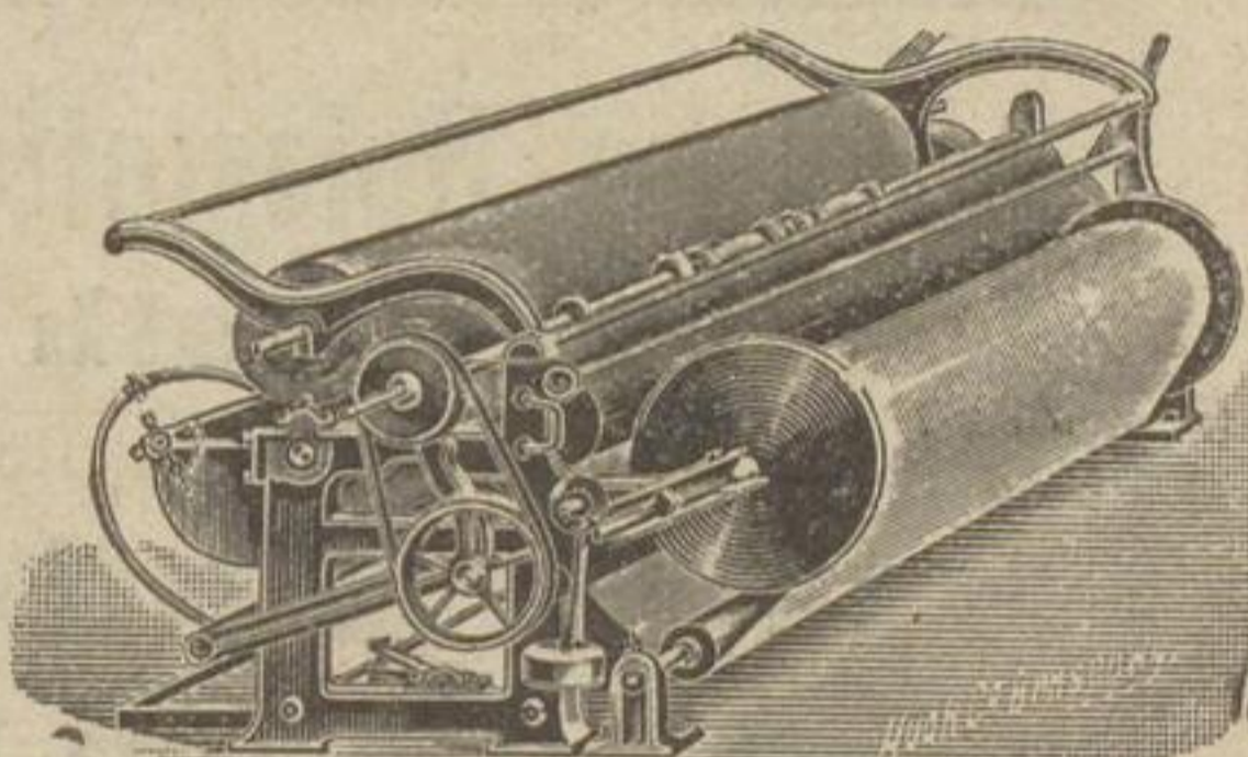
Rollen-Schneide-, Umwickel- u. Anfeucht-Maschine
