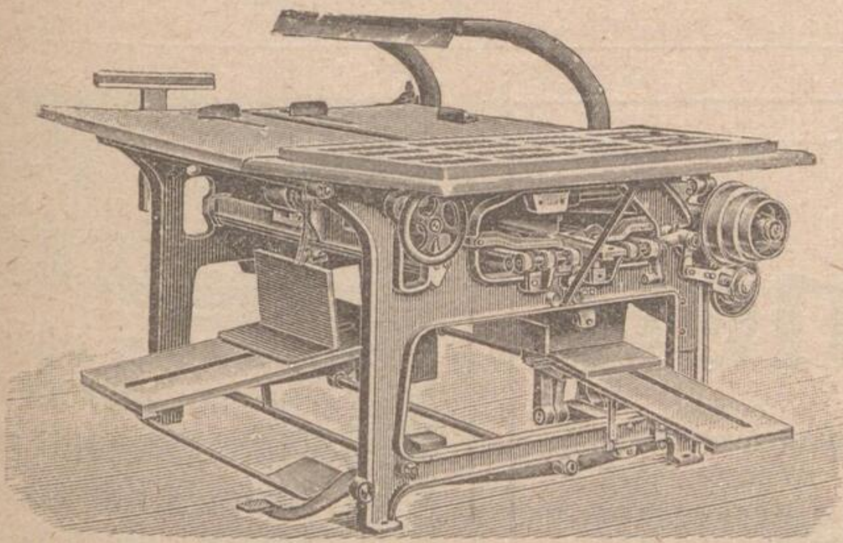
Falzmaschine für 1—4 Bruch mit der von uns zuerst gebrachten Vorrichtung zur Vermeidung von Quetschalten
