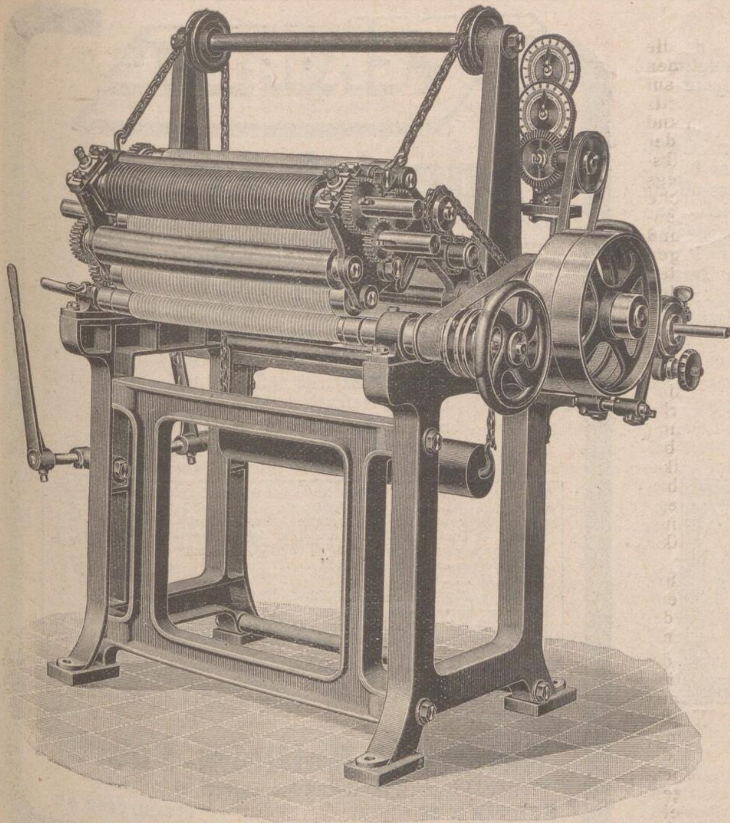
Rollenschneidmaschine
