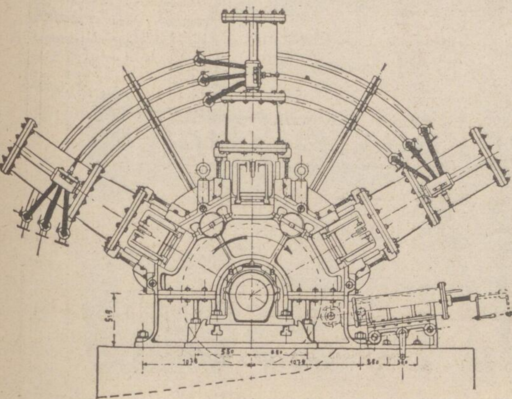
Hydraulischer Holzschleifapparat mit 3 Pressen
