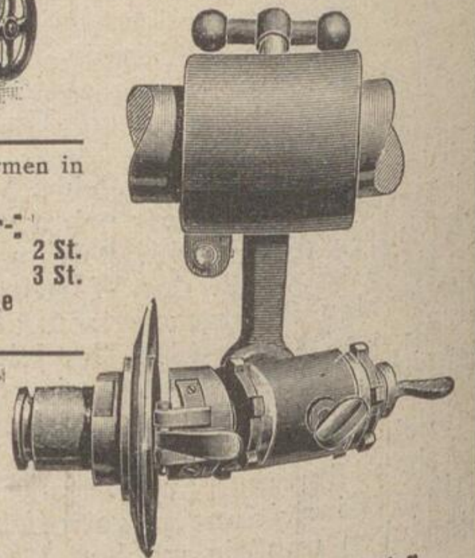
Schmidtscher Messerhalter
