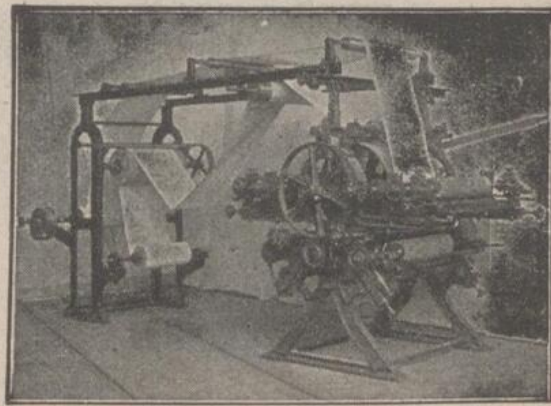
Vierfarben-Walzendruckmaschine
