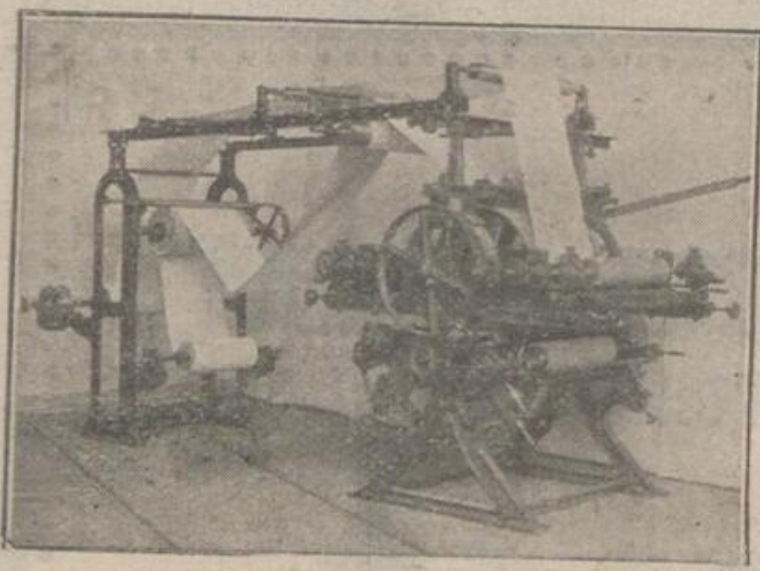
Vierfarben-Walzendruckmaschine
