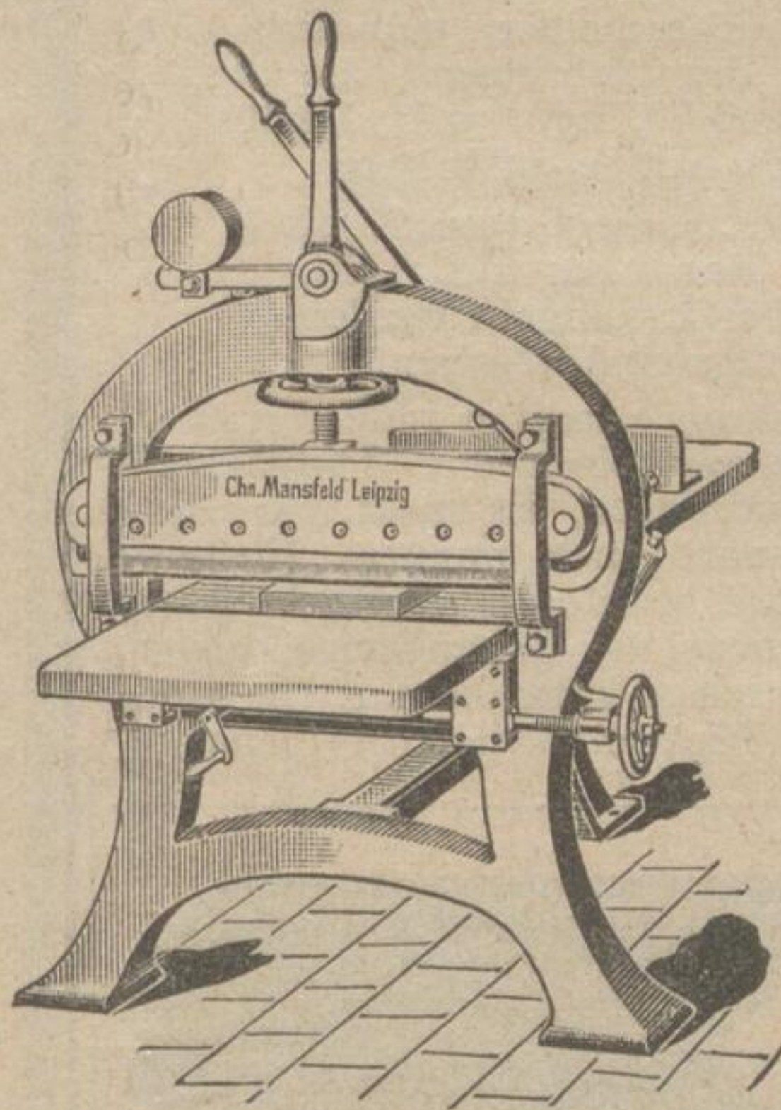
Papierschneidemaschine (Hebelsystem)
