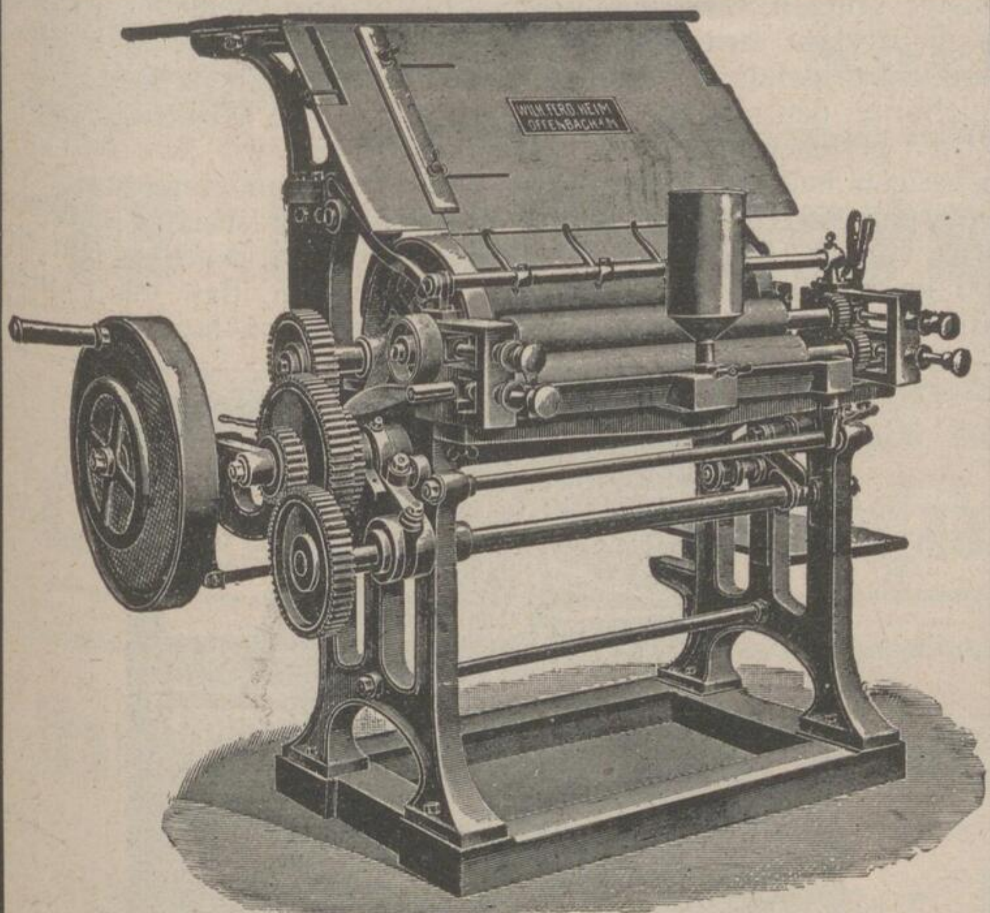
Lackier- und Gummiermaschine
