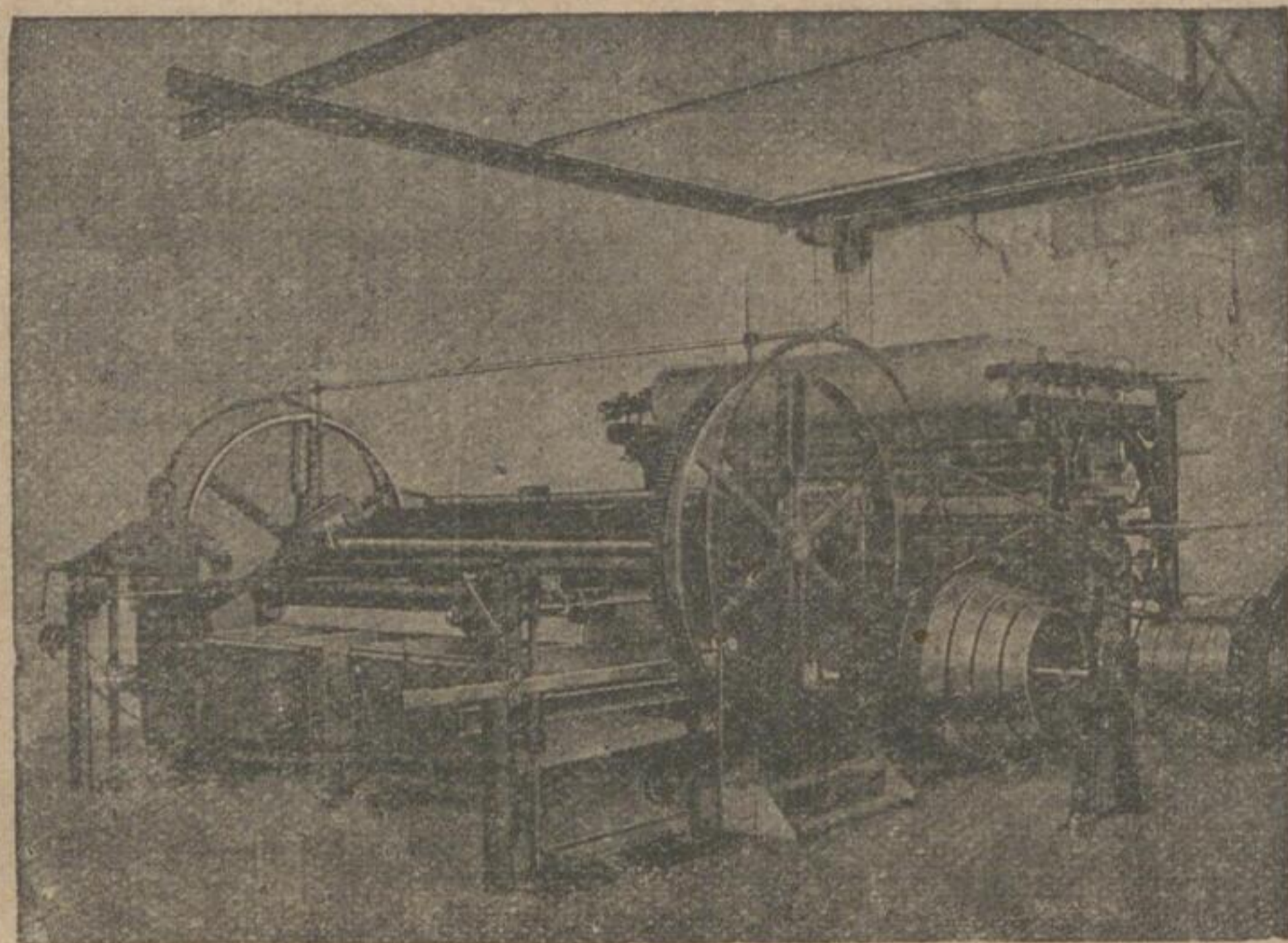
Querschneidmaschine Modell CM mit selbsttätigem Bogenableger.
