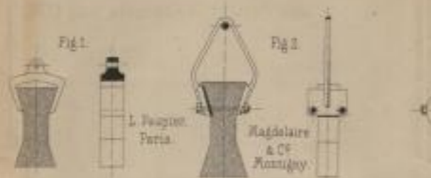
Fig. 1-5: Probestücke für Cement in No. nat. Größe
