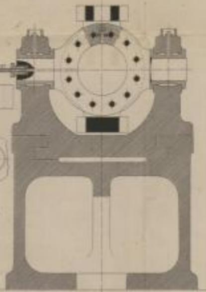
Fig. 14 Schnitt C.D. Hydraulischer Cylinder
