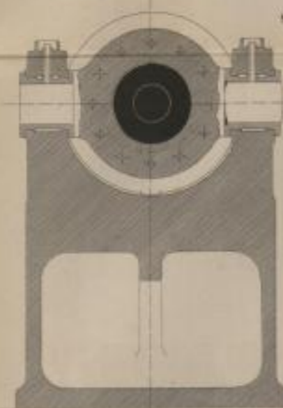
Fig. 13 Schnitt A.B. Hydraulischer Cylinder
