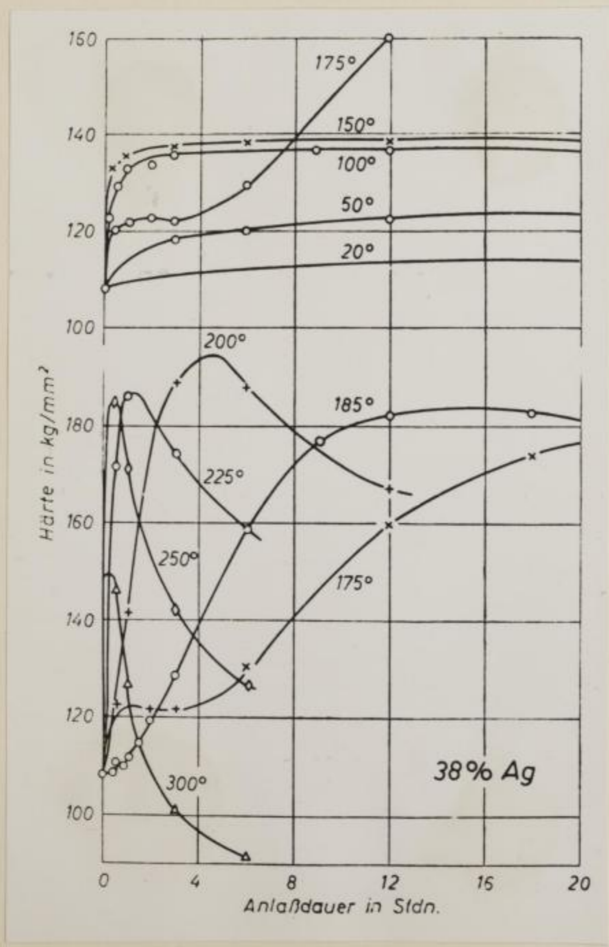
Bild 6 Abhängigkeit der Härte von der Anlaßdauer bei verschiedenen Anlaß- temperaturen für die Legierung AlAg 38 nach W. Köster und F. Braumann (24)
