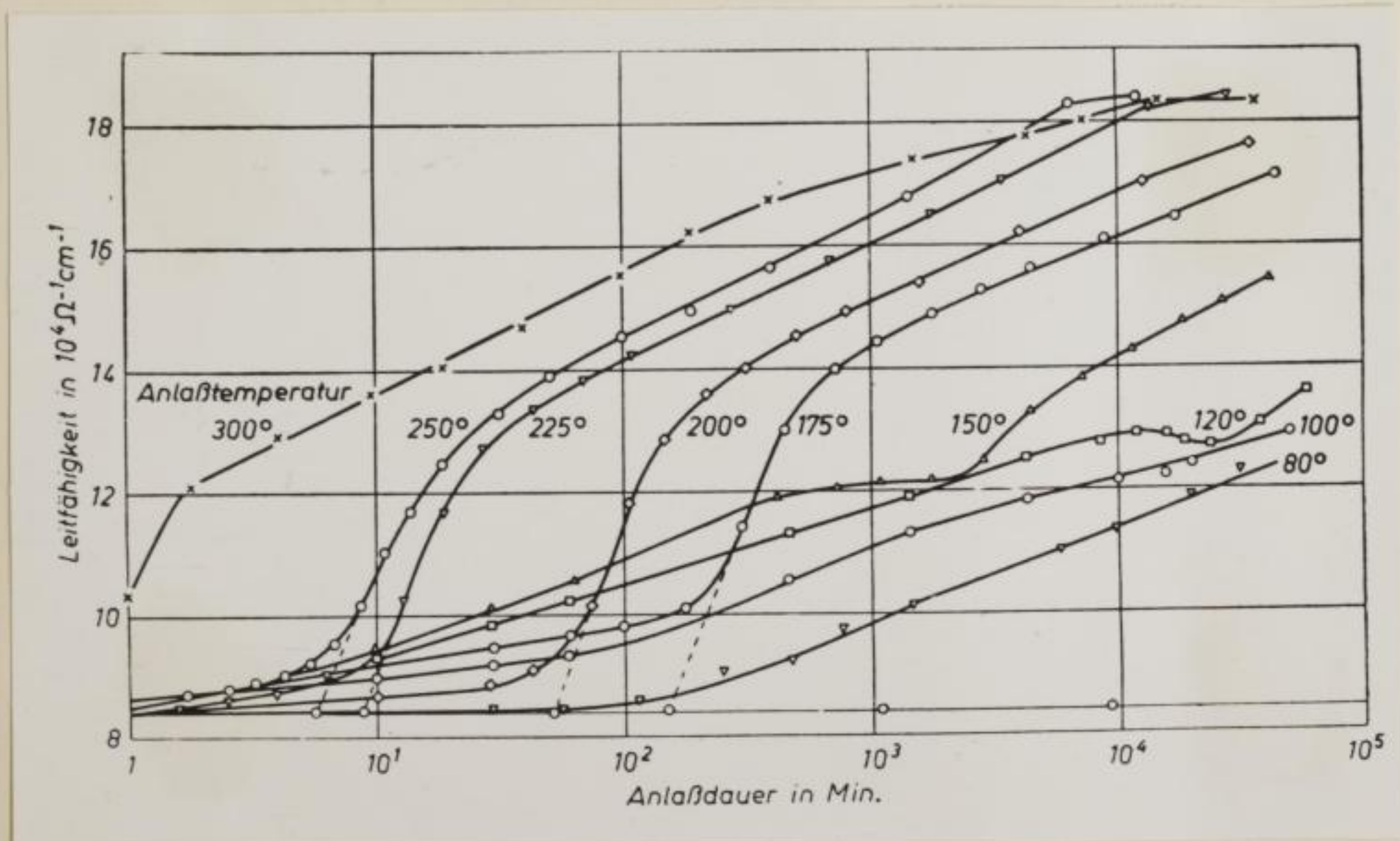
Bild 12 Änderung der elektrischen Leitfähigkeit in Abhängigkeit von der Anlaßdauer bei verschiedenen Anlaßtemperaturen nach W. Köster und Mitarbeitern (33).
