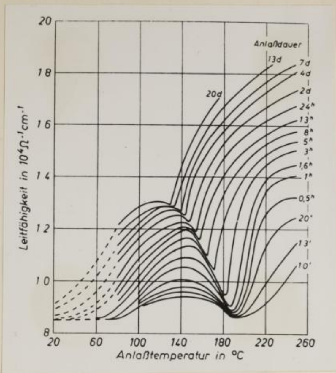
Bild 11 Änderung der elektrischen Leitfähigkeit in Abhängigkeit von der Anlaßtemperatur bei verschiedenen Anlaßzeiten nach W. Köster und Mitarbeitern (33).
