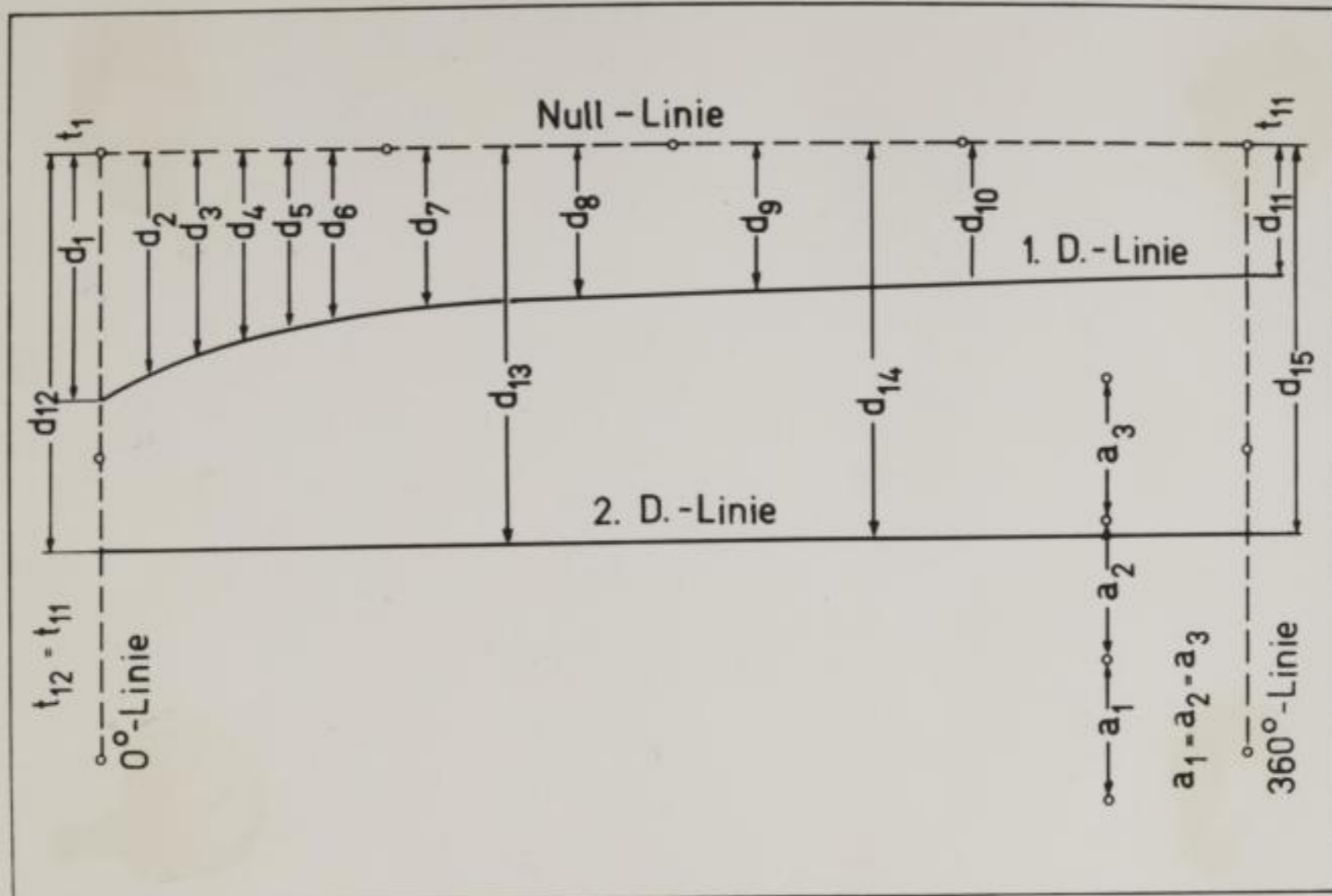
Bild 19 Schematische Darstellung der Dilatometerkurve.
