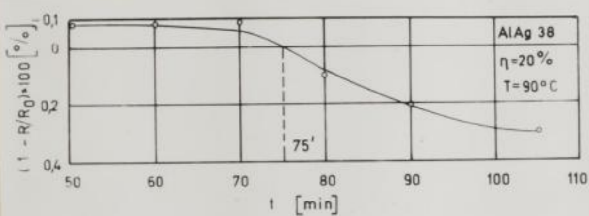
Bild 54b wie Bild 54a, jedoch T = 90^\circ\text{C} .
