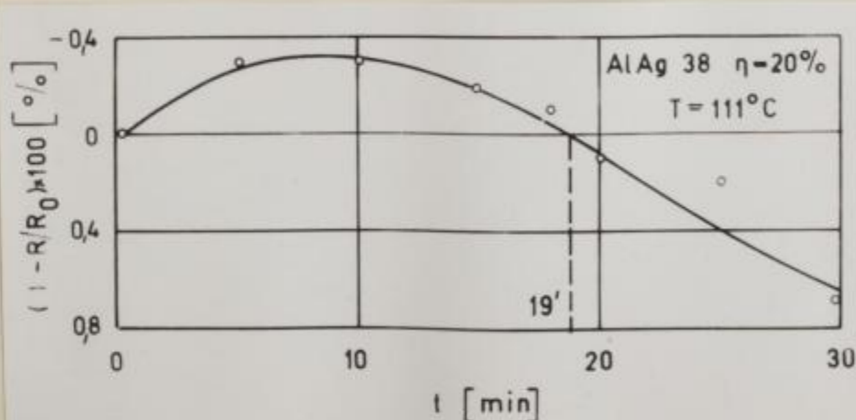
Bild 54d wie Bild 54a, jedoch T = 111^\circ\text{C} .
