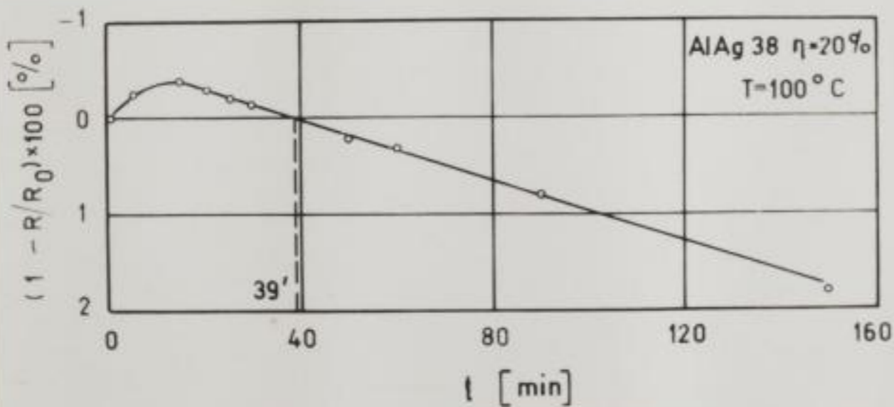
Bild 54c wie Bild 54a, jedoch T = 100^\circ\text{C} .
