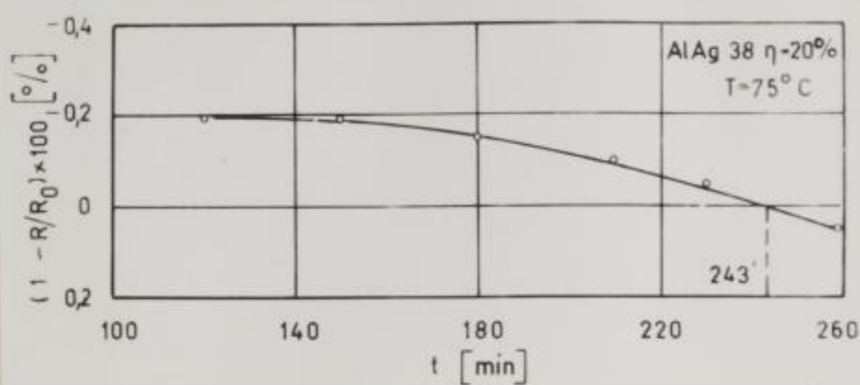
Bild 54a Relative Widerstands- änderung in Abhängig- keit von der Anlaß- dauer für \eta = 20\% , T = 75^\circ\text{C} .
