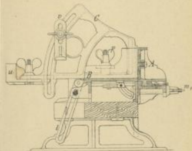
Fig. 56. Querschnitt ab.
