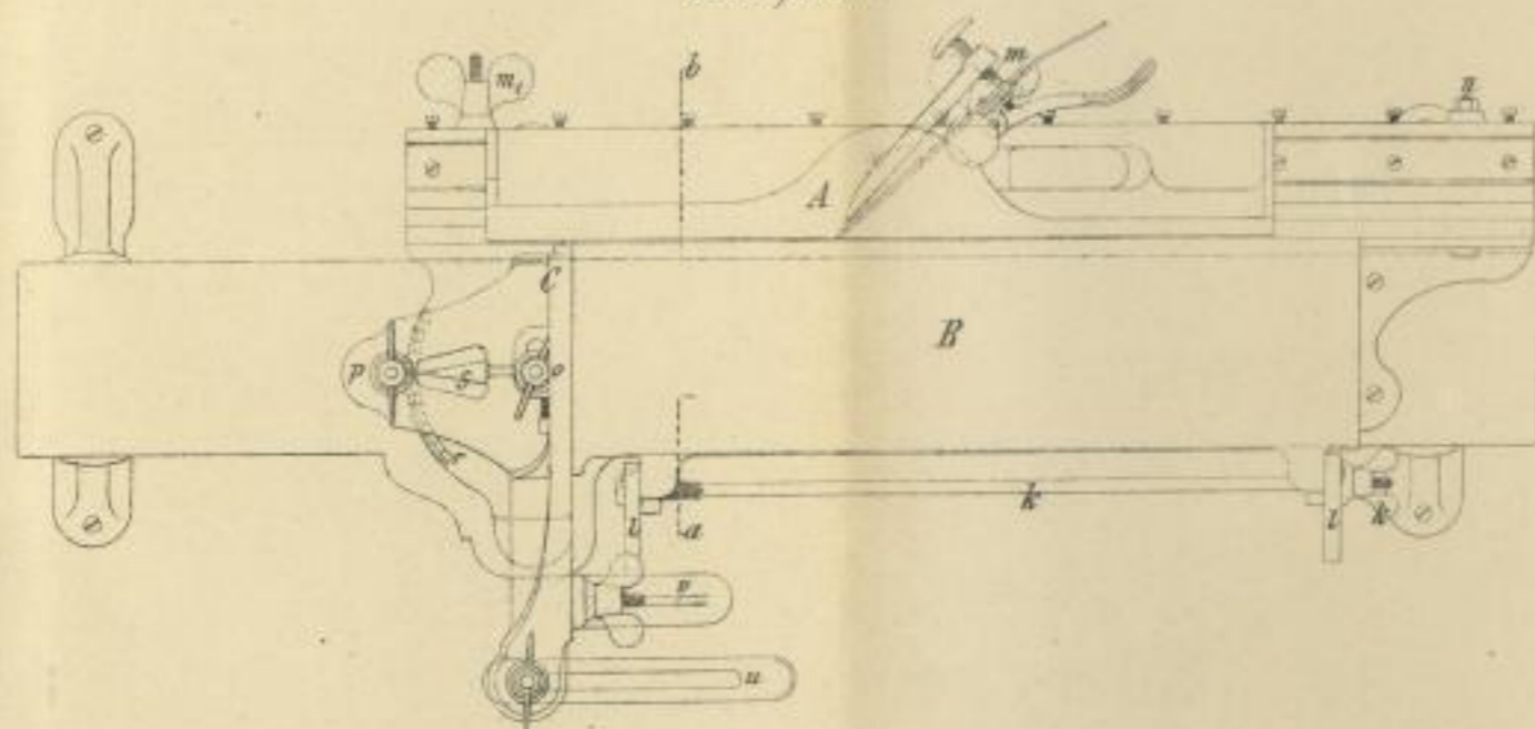
Fig. 55. Draufsicht.
