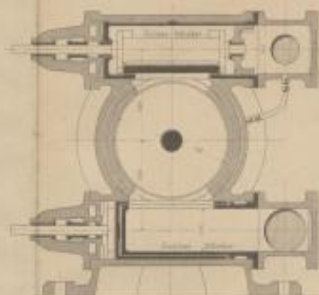
Fig. 3: Querschnitt
