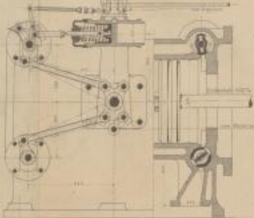
Fig. 6: Steuerung u. Zylinderschnitt
