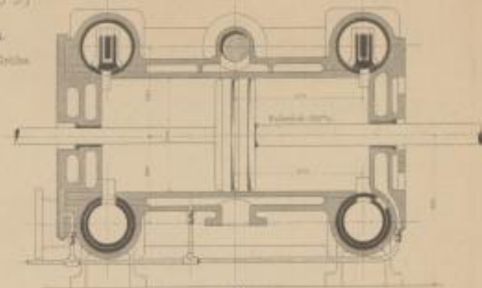
Fig. 5: Grundriss und Schnitt
