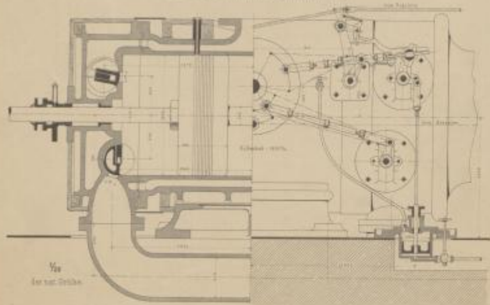
Fig. 2: Steuerung u. Zylinderschnitt
