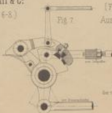
Maschine von Cail & Co (Fig. 6-8)
