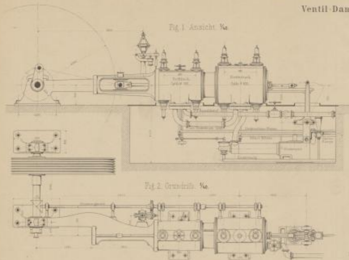
Fig. 3 Längenschnitt des Niederdruck-Cylinders
