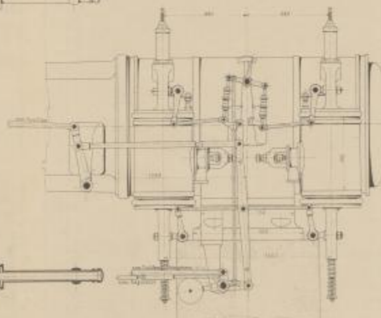
Fig 4 Ansicht der Steuerung
