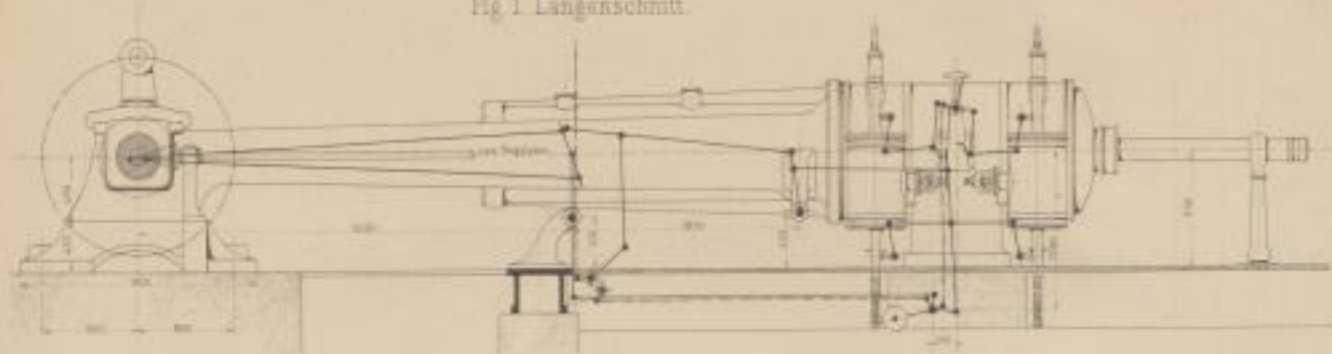
Fig 1 Längenschnitt.
