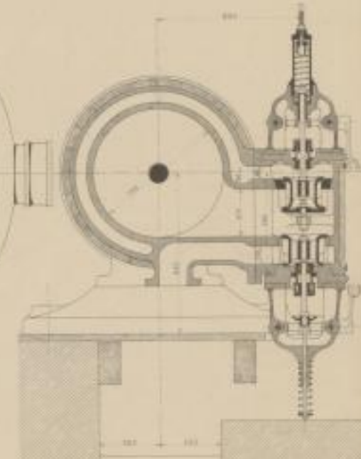
Fig 5 Zylinder-Querschnitt.
