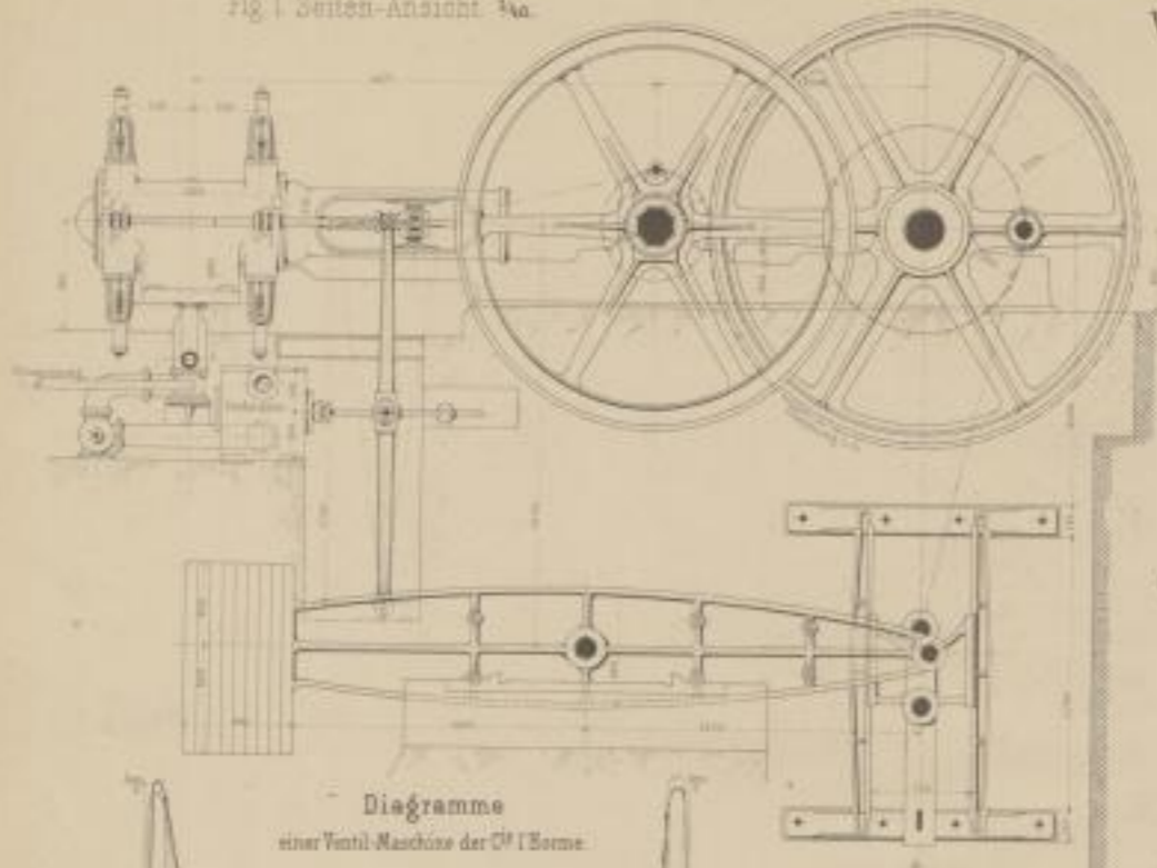
Fig. 1. Seiten-Ansicht 3/4o.
