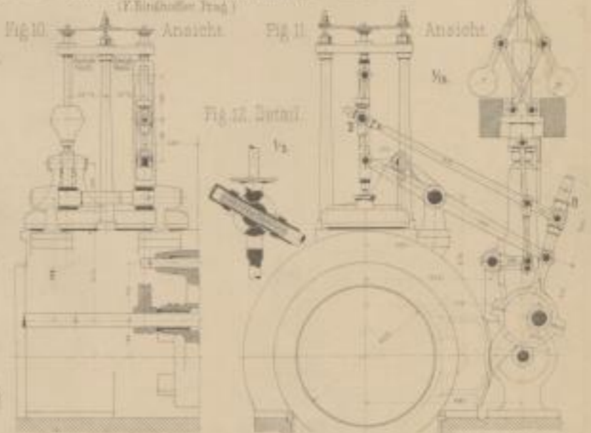
(Fig. 10-12) Umbau einer Betriebsmaschine.
