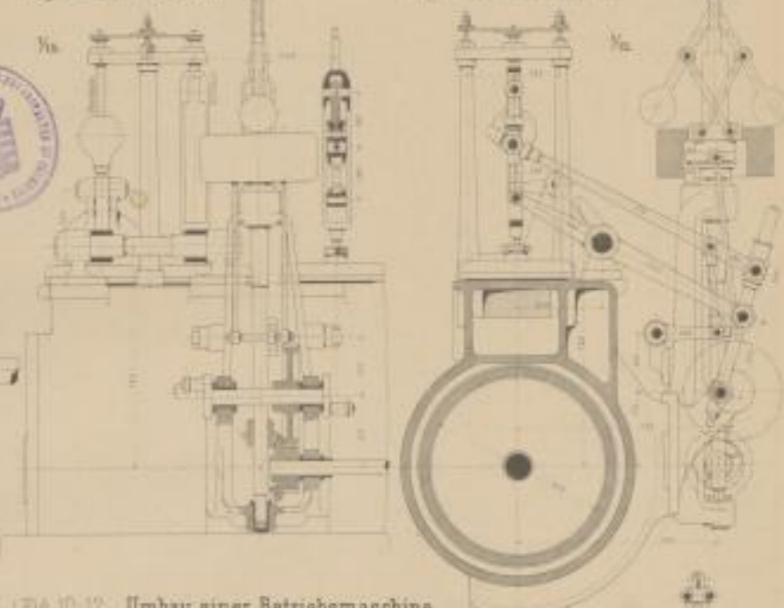
(Fig. 10-12) Umbau einer Betriebsmaschine.
