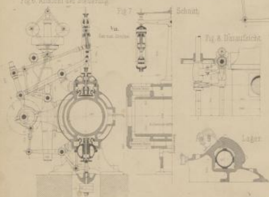
Betriebsmaschine von Dennegon in Marseille. (Fig. 6-9)
