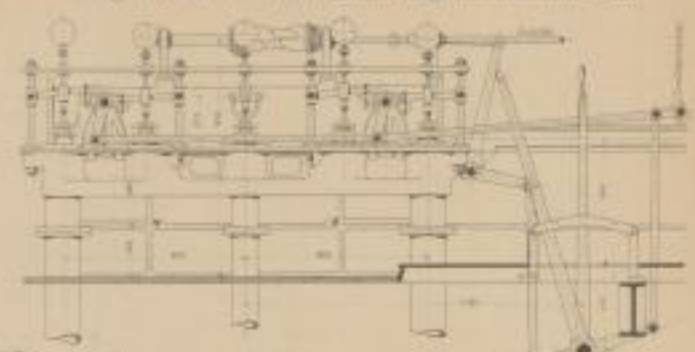
Fig. 4 Ansicht Ventil-Steuerung von Aufsemar. \frac{1}{4} .
