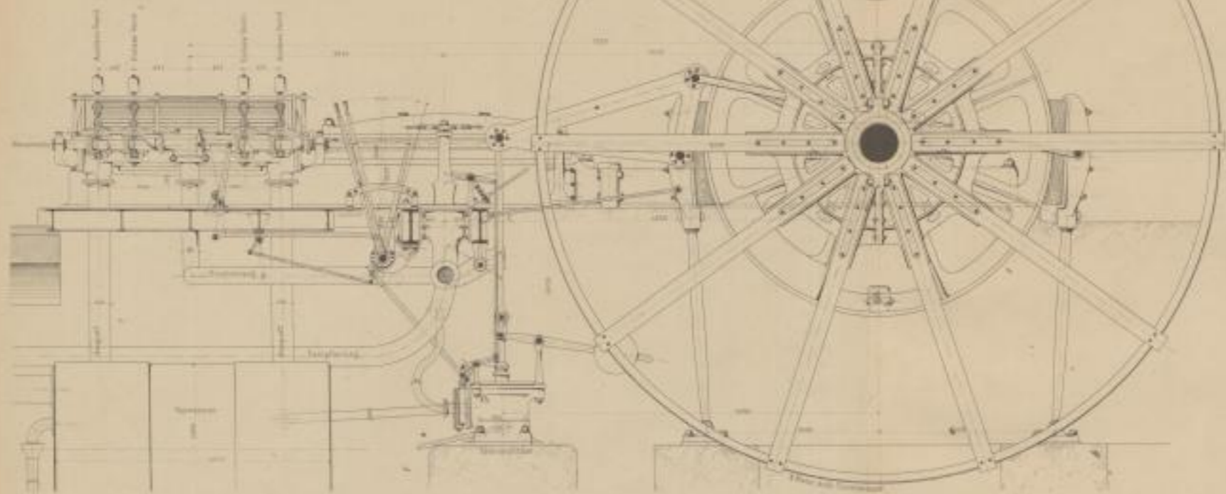
Fig. 1 Längenschnitt. \frac{1}{4} der nat. Größe.
