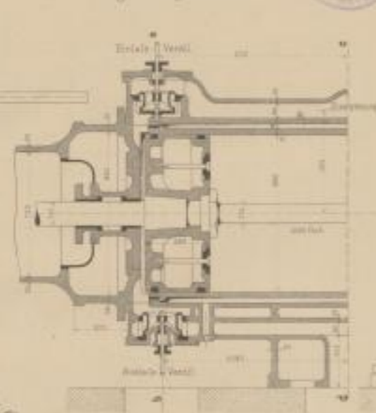
Fig. 3 Längenschnitt
