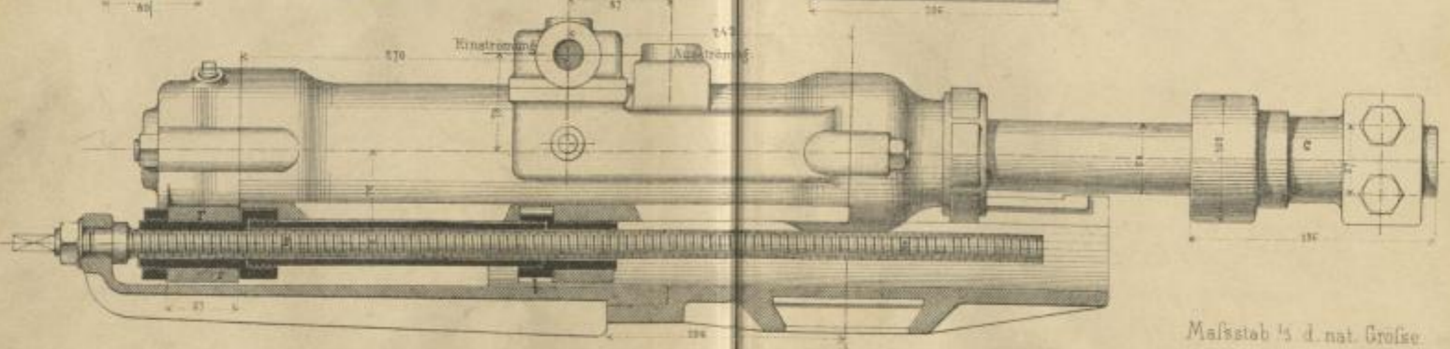
Fig. 2. Seiten-Ansicht.
