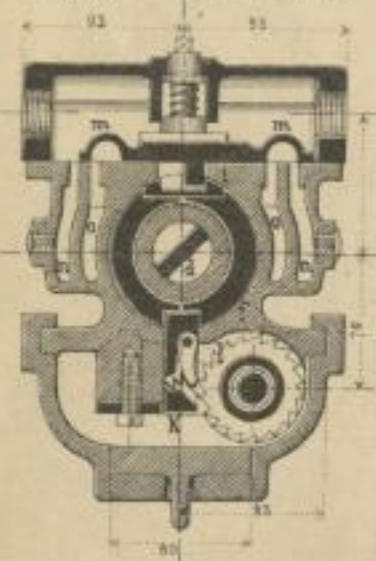
Fig. 3. Schnitt A.B.
