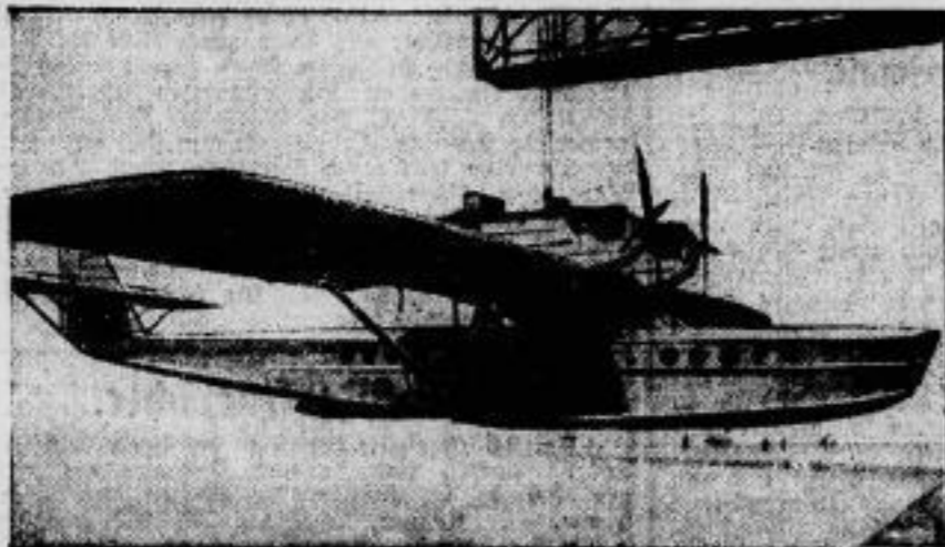
ein Flugboot, das besondere Bedeutung für künftige Ozeanflüge haben wird. Das Flugboot hat ein Fassungsvermögen von 20 Personen. — Unser Bild zeigt den Dornier-Super-Dol an seiner Hängvorrichtung in der Friedrichshafener Werft.
