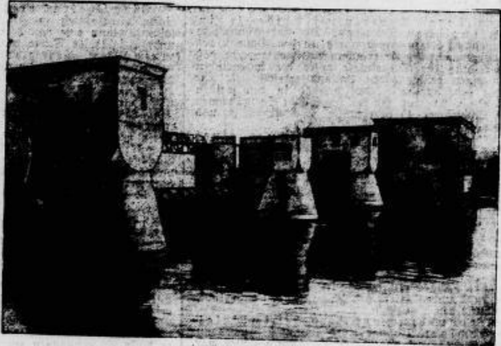
Gärten der Arbeit. Das riesige Wasserwerk der Großfläranlage Hengsten am Fuße der Hohen- Isenburg , die das Wasser der Ruhr zur Schlammablagerung in einem großen See führt. Mit dem Wehr ist eine Wasserkraftanlage verbunden, die eine Tages- leistung von 48000 Kilowattstunden ergibt. Der gesamte Bau, der im Früh- jahr 1926 begonnen wurde, soll im nächsten Jahr fertiggestellt sein.
