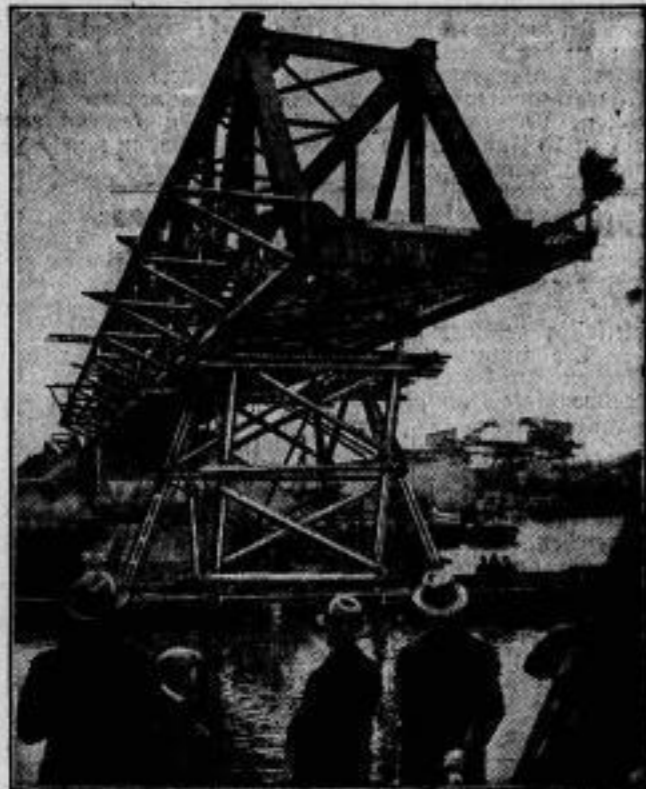
Moderner Brückenbau. Beim Bau einer neuen Brücke über den Spandauer Schiffsfahrtskanal bei Berlin wurde die Brücke auf dem Zufahrtsdamm vollständig montiert und konnte dann im Verlauf eines einzigen Tages über den Kanal gelegt werden. Der dort sehr lebhafte Schiffsverkehr wurde dadurch nur für kurze Zeit unterbrochen. Unser Bild zeigt, wie die Brücke, mit dem einen Ende auf einem Kahn aufliegend, langsam über das Wasser geschoben wird.
