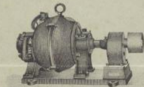
Reduktions-Kupplungen zur Verminderung der Geschwindigkeiten bei Elektromotoren.
