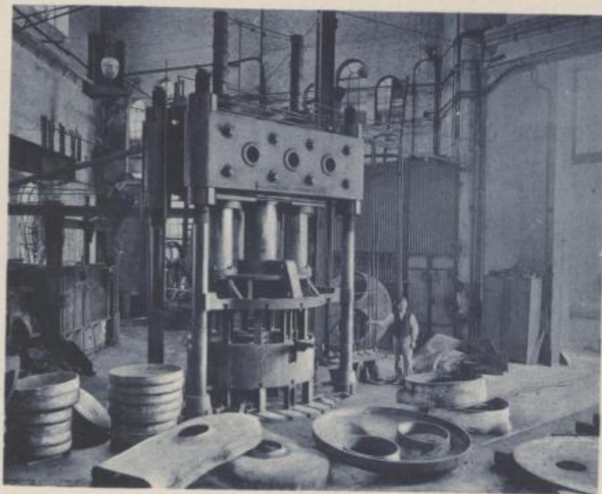
Hydraulische Kumpelpresse.
