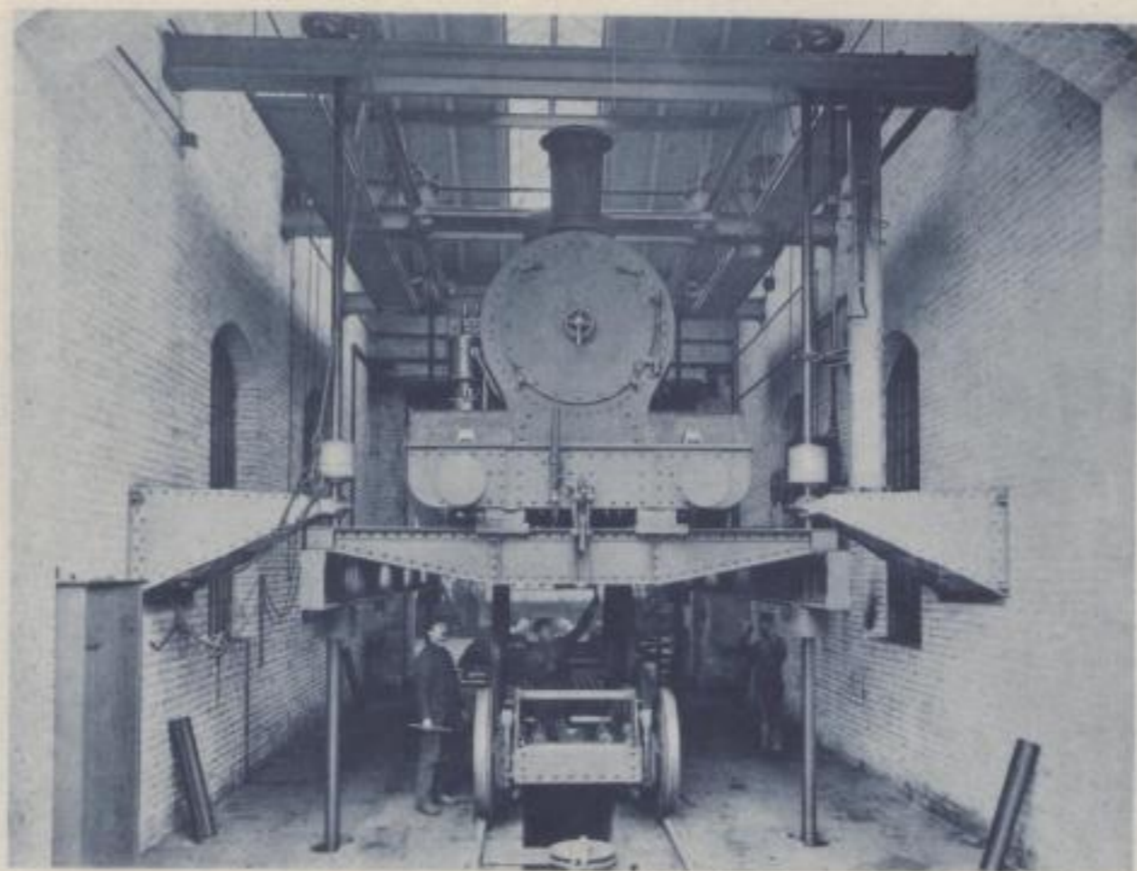
Electrische Hebevorrichtung für Locomotiven.
