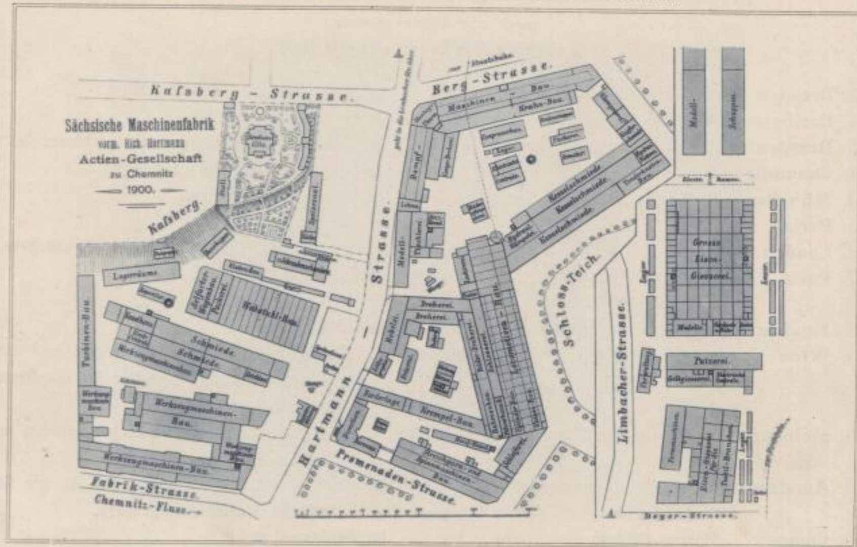
Grundriss der Fabrikanlagen.
