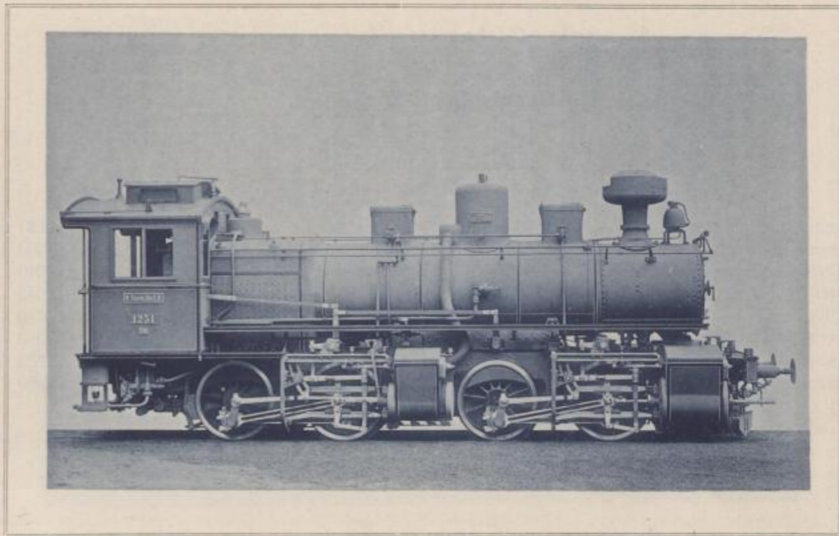
Sächsische Maschinenfabrik vorm. Rich. Hartmann, A.-G. zu Chemnitz.
