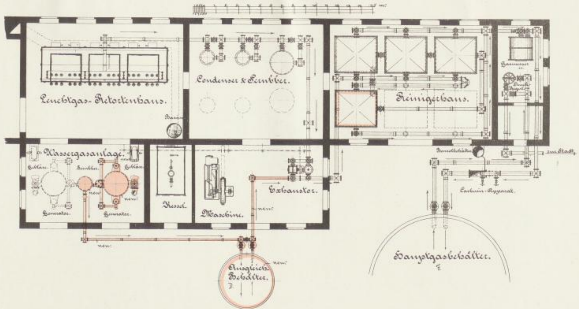
Erweiterung einer Steinkohlengasanlage durch Wassergas, carburirt mittels Benzol.
