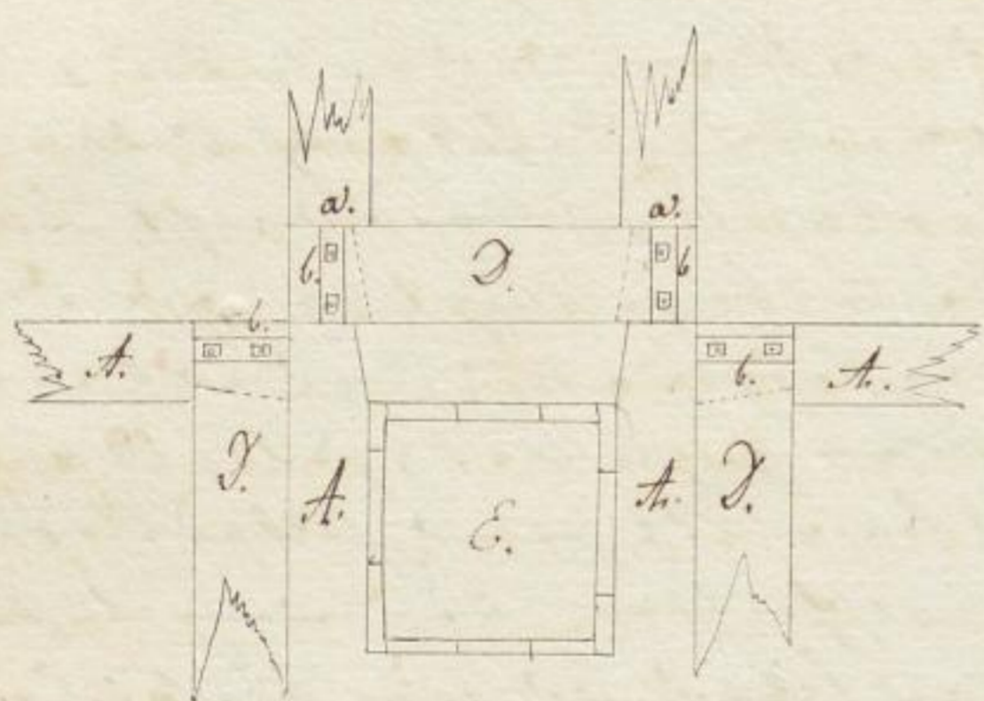
Äußere Ansicht des Aufbaus der Viertelbleche auf dem Gerüst (Tafel 1. äussere Ansicht davon)
