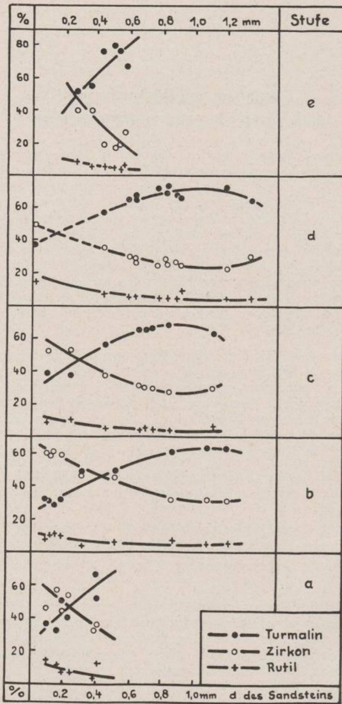
Bild 16. Diagramm der Schwermineralverteilung in der Kornklasse 0,1–0,05 mm für die Proben der turonen Sandsteinstufen a bis e im Elbsandsteingebirge. Kornanzahl Turmalin + Zirkon + Rutil = 100 %. Nach SCHEIDHAUER (1939, S. 485)
