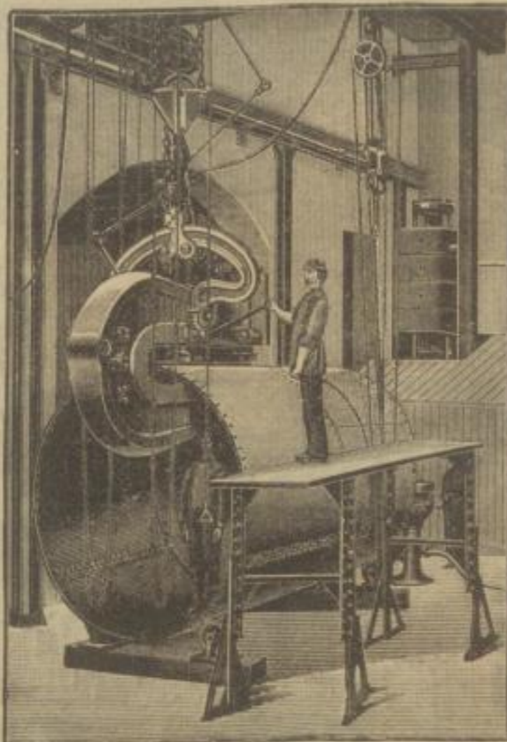
Hydraulische Nietanlage.
